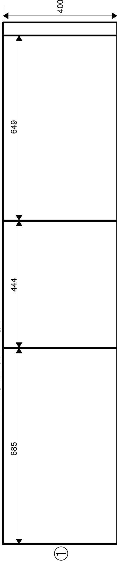
18 x 400 x 1820 パイン集成材 2枚
